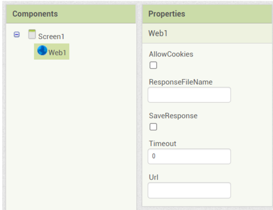
Ekran Görüntüsü 43. Web Nesnesi Özellikler Bölümü
