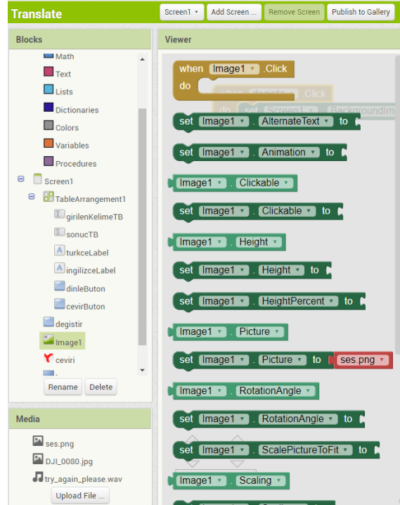
Ekran Görüntüsü 22.Blocks sekmesinden resim ekleme ve yönetme
