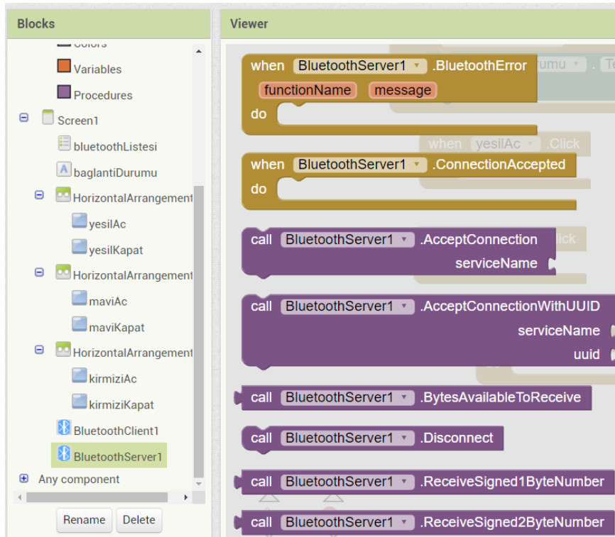
Ekran Görüntüsü 48. Bluetooth Sunucu Bloklar Ekranı
