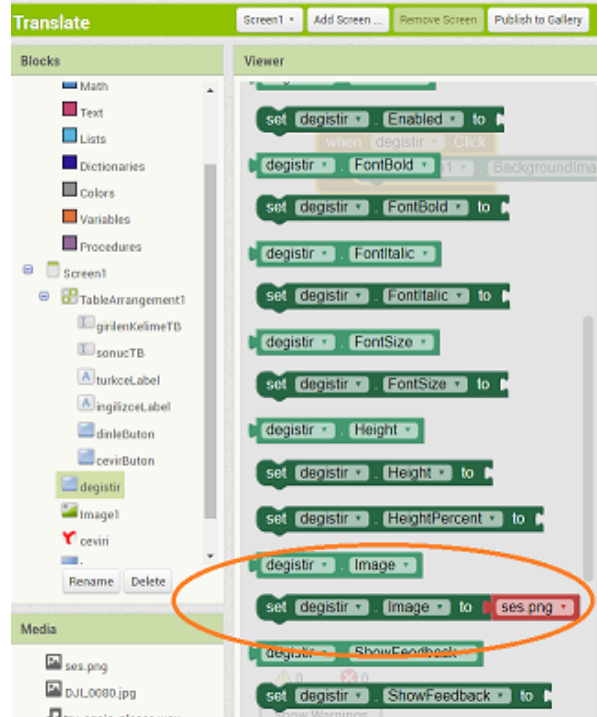
Ekran Görüntüsü 24. Blocks sekmesinden buton arka plan resmi ekleme
