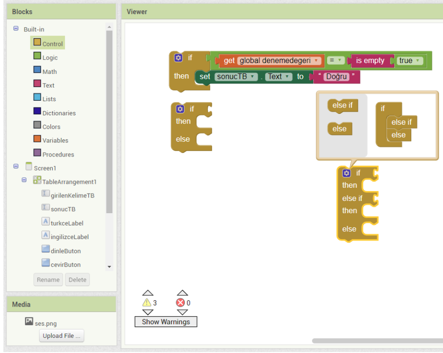
Ekran Görüntüsü 33. Örnek koşul (if, else, then) yapısı
